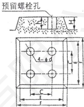
硬性联接基础图
