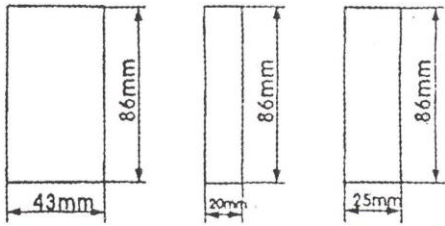
SD 型隔振垫 0.5 基本块尺寸
