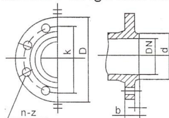
法兰图 Flange Drawing
